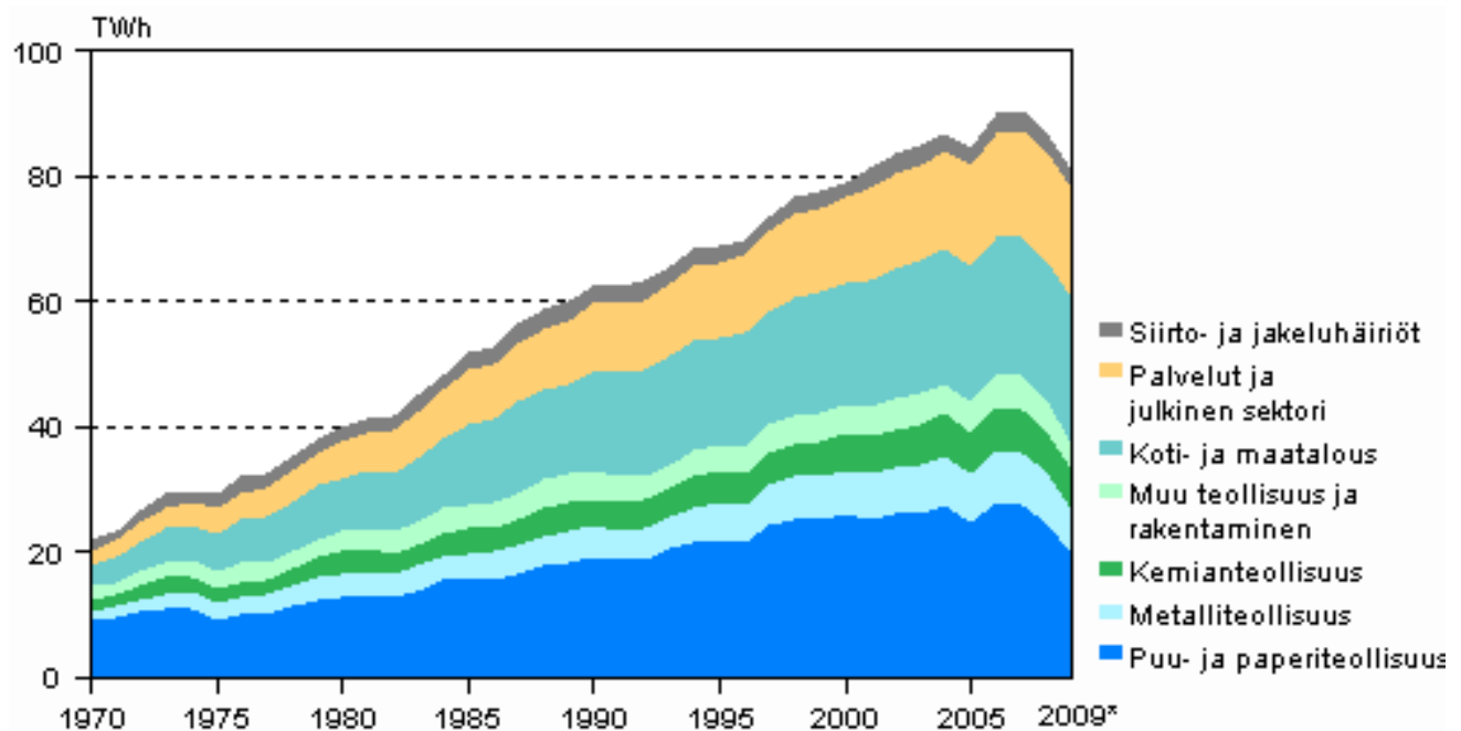
Kuva. Sähkön kulutus sektoreittain (Lähde: Tilastokeskus).
